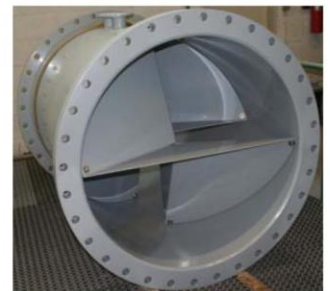
Mischer DN 1200 mit Rilsanbeschichtung
