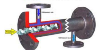
Wärmetauscher für hochviskose Medien mit Wendelmischelementen
