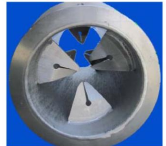
verstopfungsfreier Statischer Mischer
