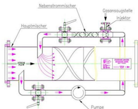
Dispergiergerät
